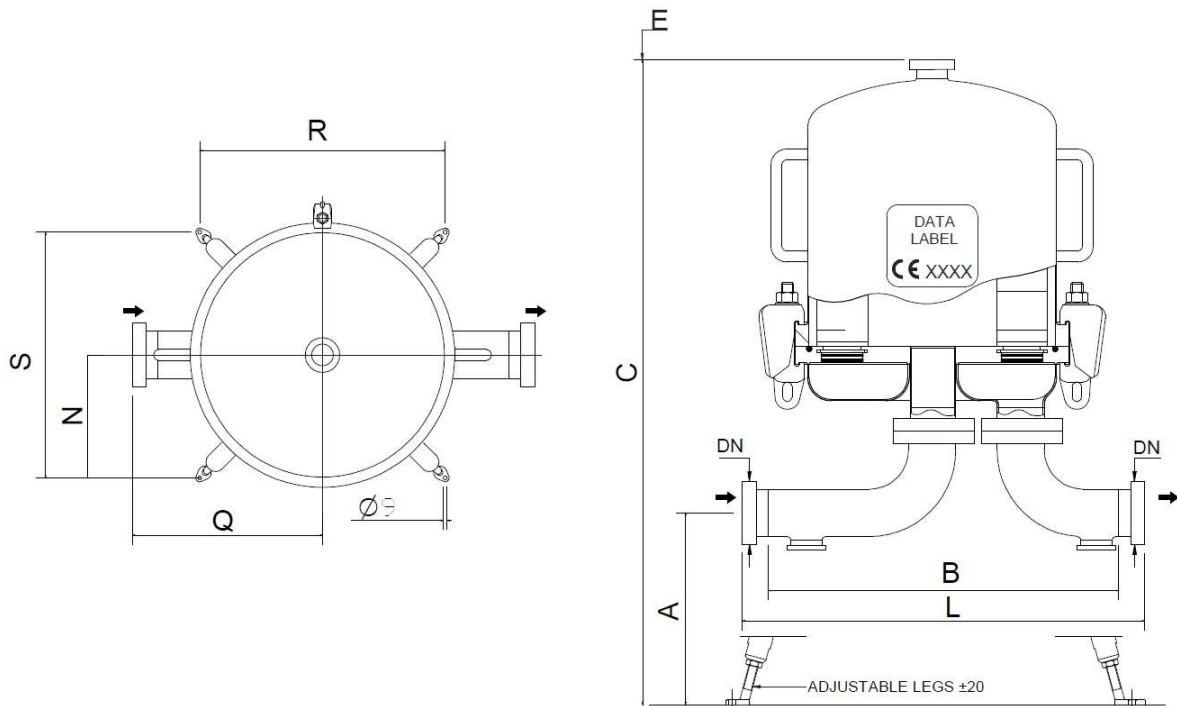
Dimensions PF-EG 0320-3040
